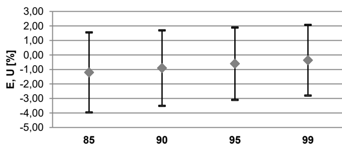
ERROR E INCERTIDUMBRE EXPANDIDA SATURACIÓN PARCIAL DE OXÍGENO
