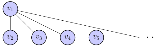
Figura 1.1.10: Un grafo infinito que no es localmente finito
