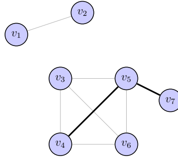
Figura 1.1.13: Un camino entre v_4 y v_7
