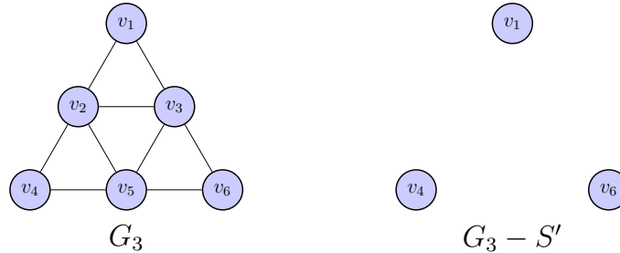
Figura 1.1.18: G_3 y G_3 - S'
