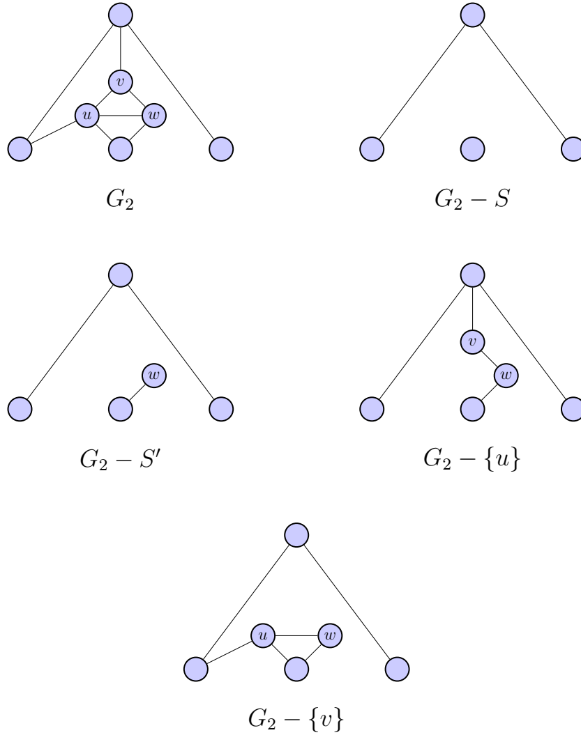
Figura 1.1.20: Efecto de eliminar subconjuntos de vértices en G_2
