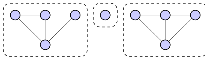
Figura 1.1.16: Un grafo con tres componentes
