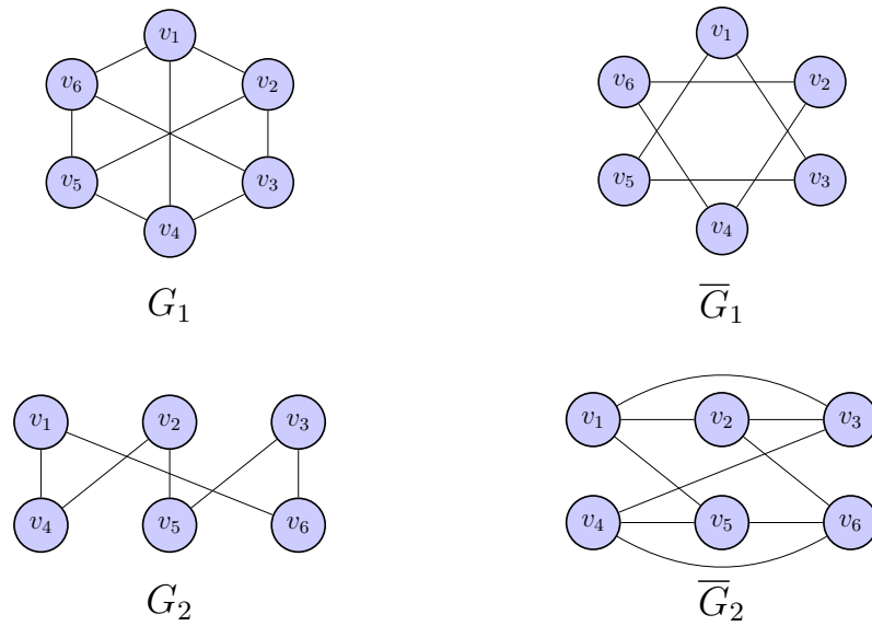
Figura 1.1.21: Grafos y sus complementos
