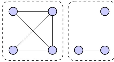
Figura 1.1.15: Un grafo con dos componentes
