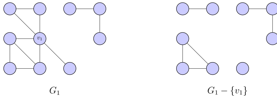
Figura 1.1.19: Un vértice de corte
