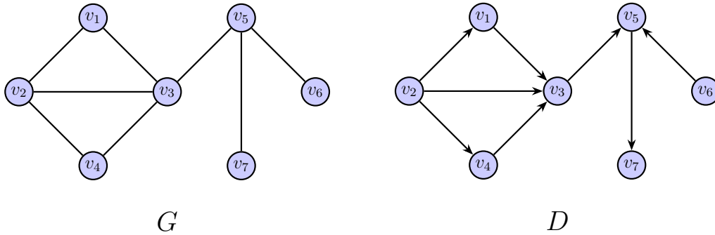
Figura 1.1.4: D es una orientación de G
