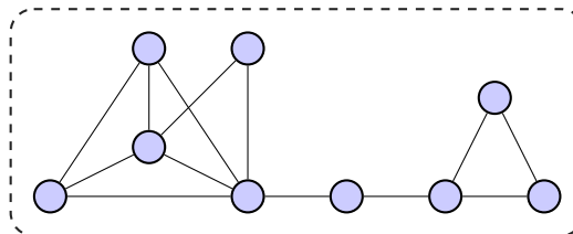
Figura 1.1.14: Un grafo con una componente
