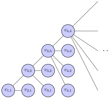
Figura 1.1.9: Un grafo infinito localmente finito
