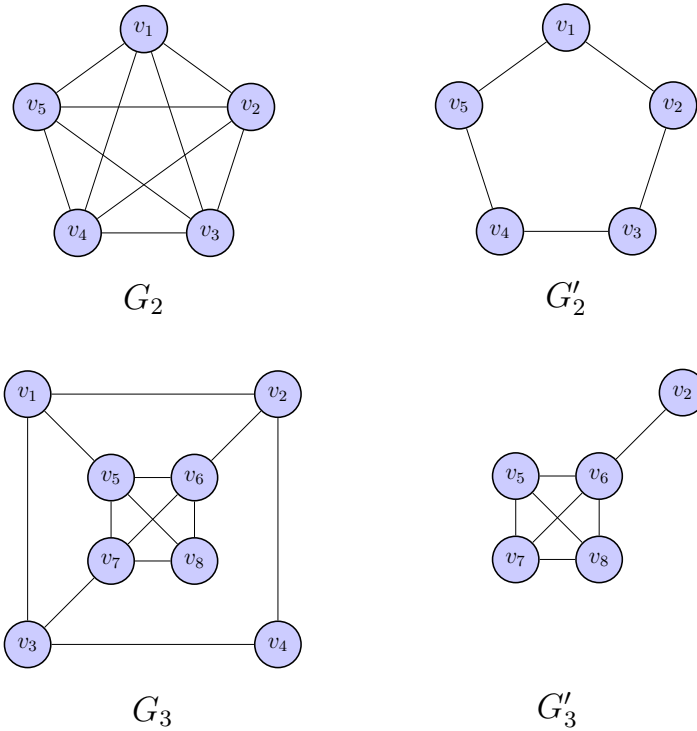
Figura 1.1.6: Ejemplos de contenencia de grafos
