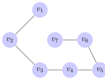
Figura 1.1.6: P^6 = v_1v_2v_3v_4v_5v_6v_7
