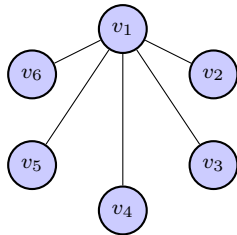
Figura 1.1.1: Ejemplos de grafos sobre V
