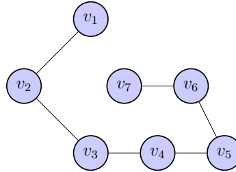
Figura 1.1.12: P^6 = v_1v_2v_3v_4v_5v_6v_7
