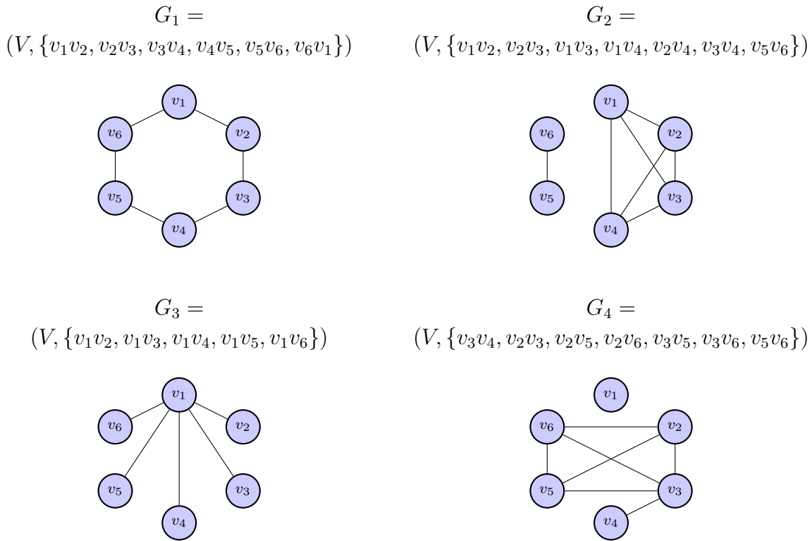
Figura 1.1.6: Ejemplos de grafos sobre V
