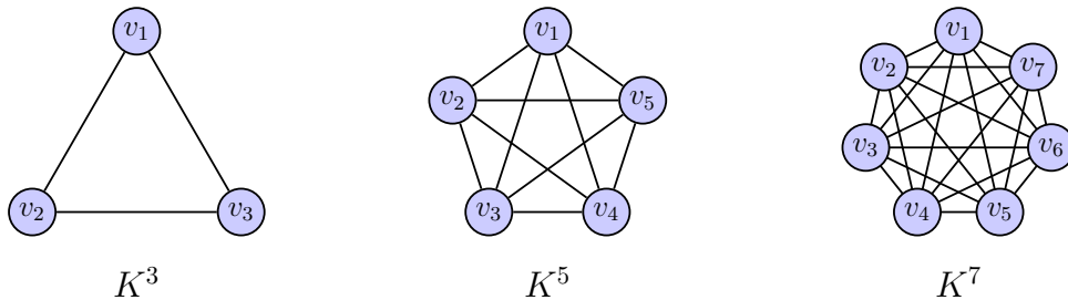
Figura 1.1.25: Ejemplos de grafos completos
