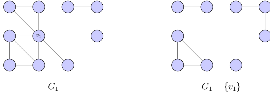
Figura 1.1.20: Un vértice de corte
