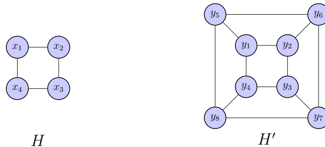
Figura 1.1.33: H y H'
