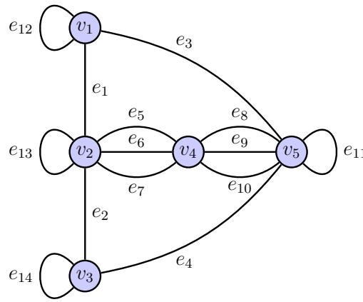
Figura 1.1.4: Un multigrafo
