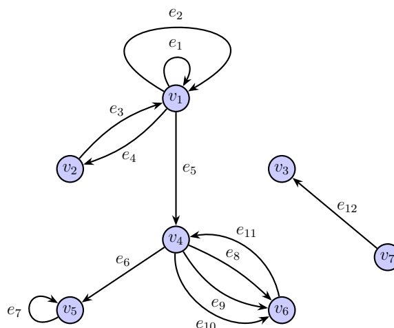
Figura 1.1.3: Un grafo dirigido
