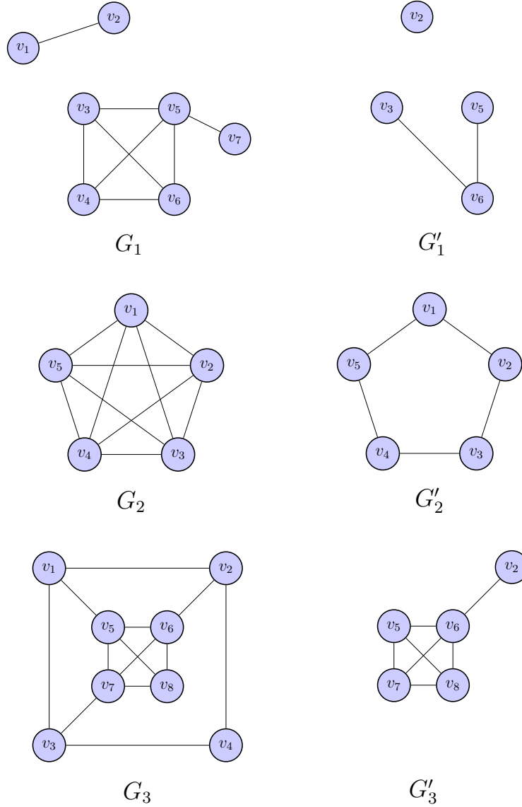
Figura 1.1.4: Ejemplos de contenencia de grafos
