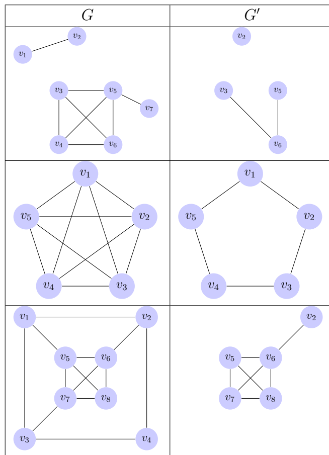
Cuadro 1.1: Ejemplos de contención de grafos
