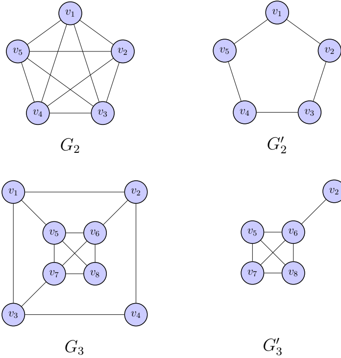
Figura 1.1.4: Ejemplos de contenencia de grafos
