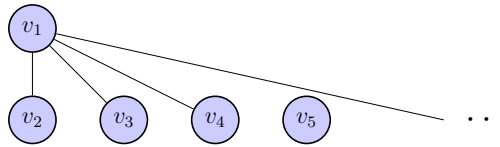
Figura 1.1.8: Un grafo infinito que no es localmente finito
