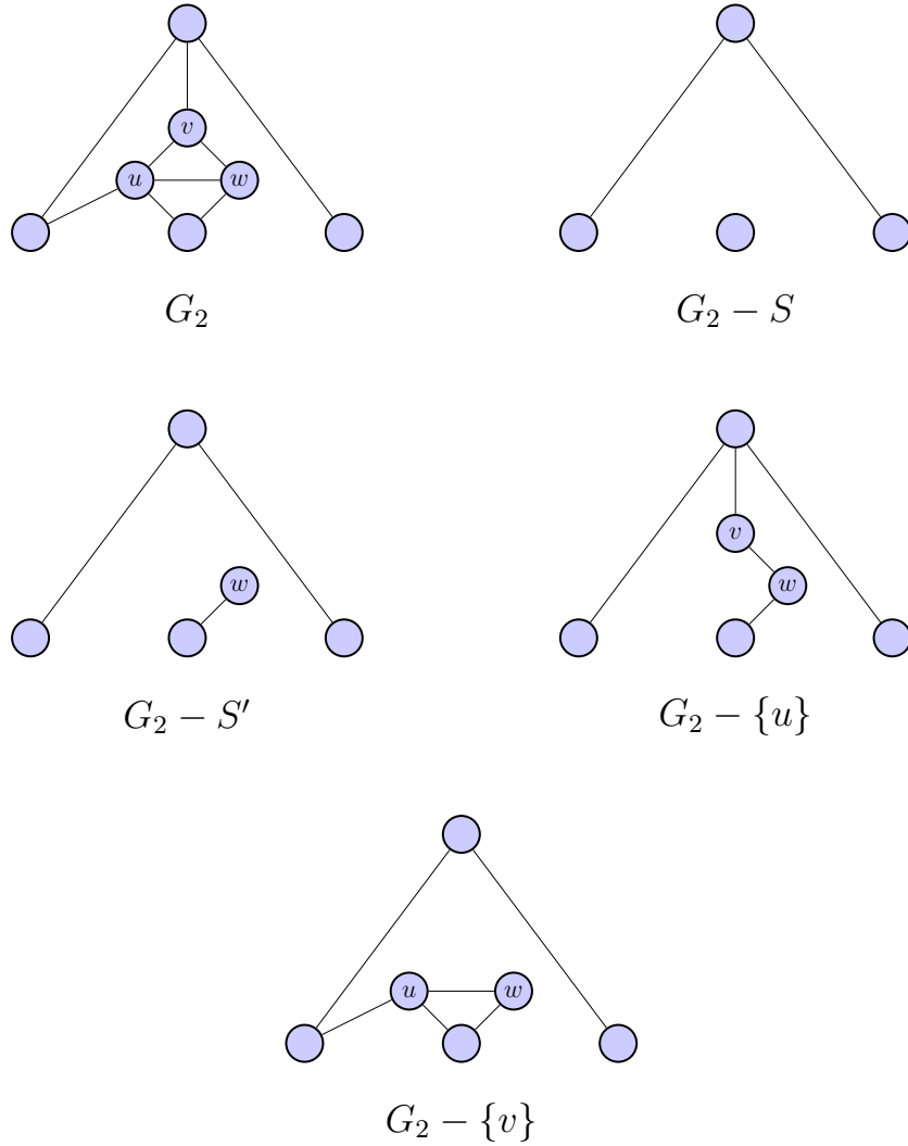
Figura 1.1.18: Efecto de eliminar subconjuntos de vértices en G_2
