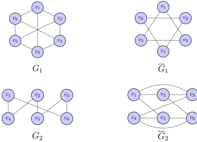
Figura 1.1.19: Grafos y sus complementos
