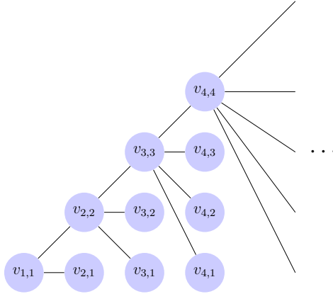
Figura 1.4: Un grafo infinito localmente finito
