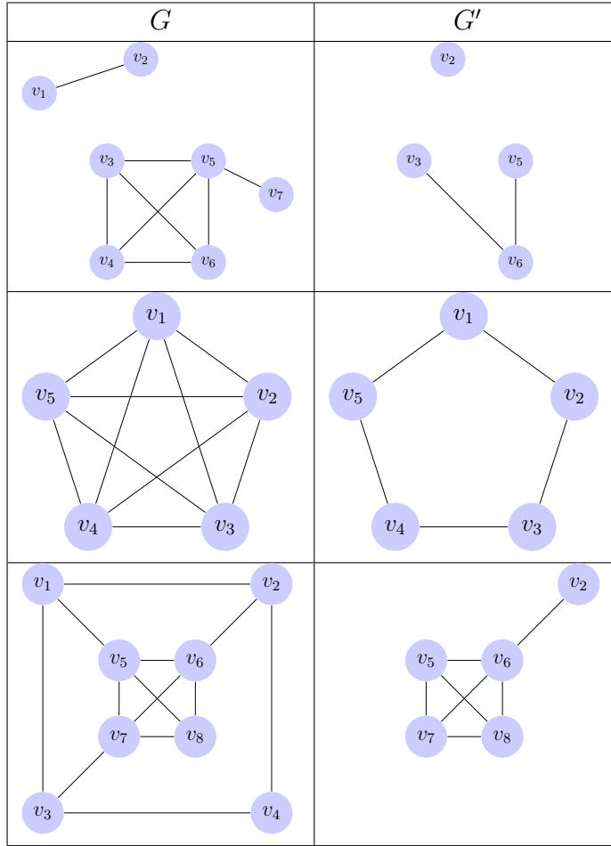
Cuadro 1.1: Ejemplos de contenencia de grafos
