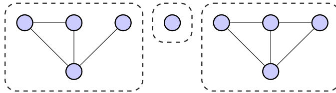
Figura 1.1.11: Un grafo con tres componentes
