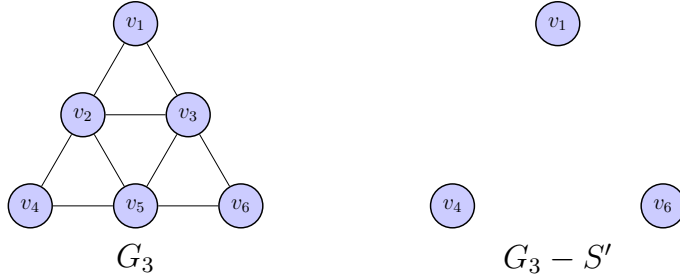
Figura 1.1.13: G_3 y G_3 - S'
