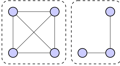
Figura 1.1.10: Un grafo con dos componentes
