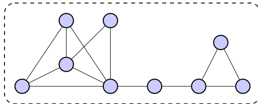
Figura 1.1.9: Un grafo con una componente
