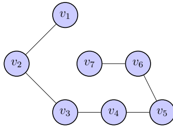
Figura 1.1.12: P^6 = v_1v_2v_3v_4v_5v_6v_7
