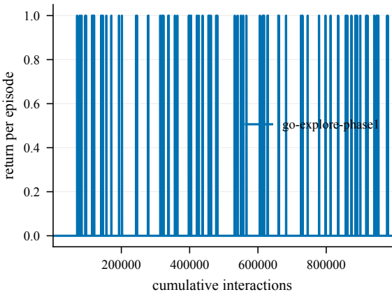
Return -- EpicChase1-60@4
