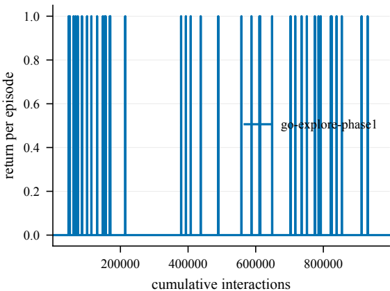
Return -- EpicChase2-70@3
