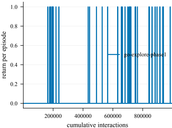
Return -- EpicChase2-70@4
