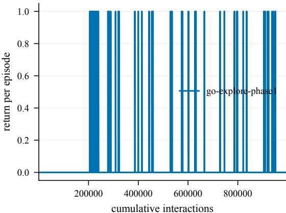
Return -- EpicChase2-70@5
