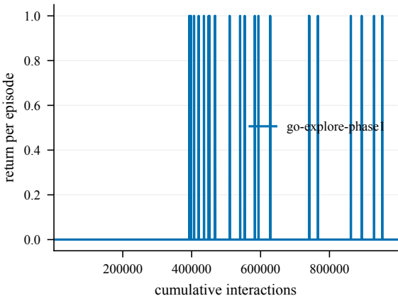
Return -- EpicChase4-90@3
