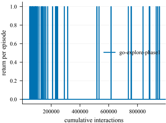
Return -- EpicChase6-110@10
