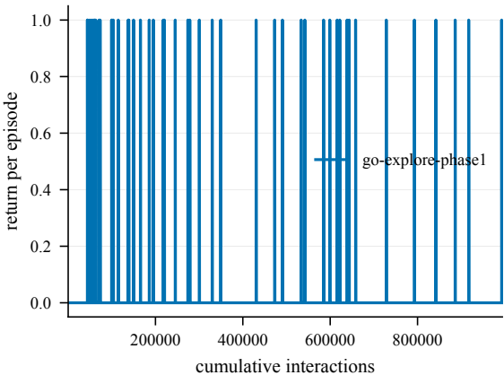
Return -- EpicChase6-110@23
