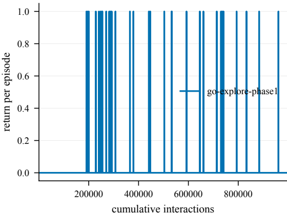
Return -- EpicChase6-110@5
