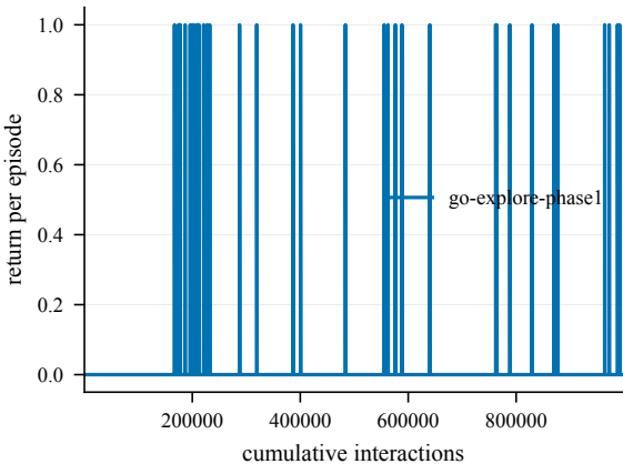
Return -- EpicChase6-110@7
