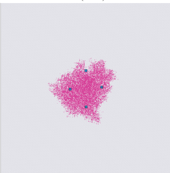
TE (none)
