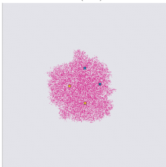
TE (ricci)
