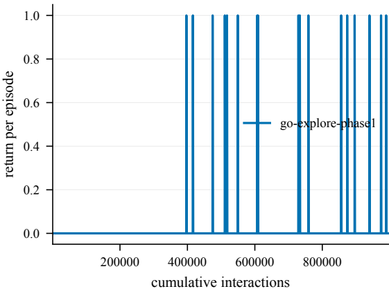
Return -- Bottleneck6-100@4000
