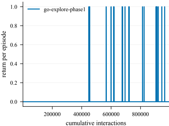
Return -- Bottleneck6-200@4000
