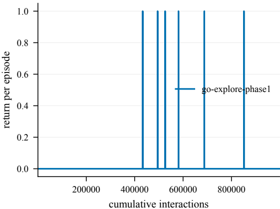
Return -- ChamberCount8-100@4000
