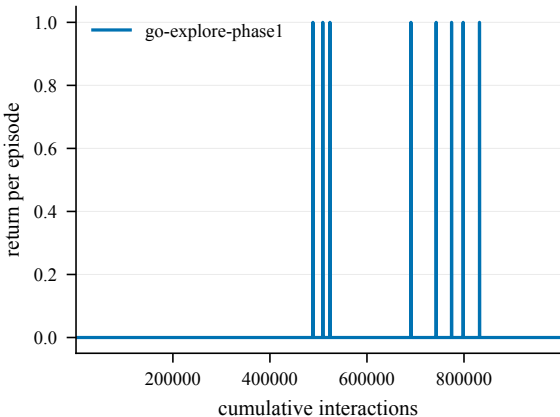
Return -- Chambers2-100@4000
