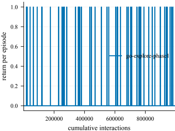
Return -- Chambers2-50@4002
