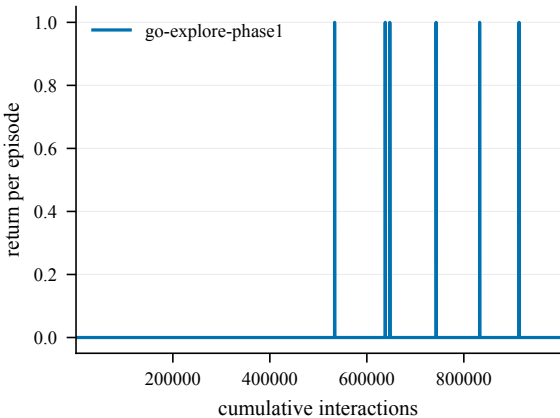
Return -- Decoys0-100@4002
