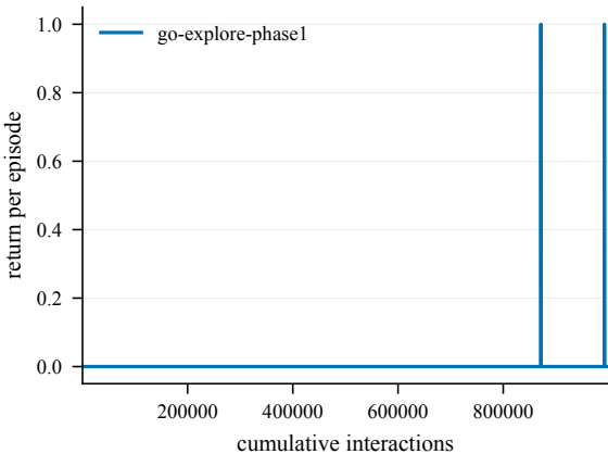
Return -- Decoys1-100@4001
