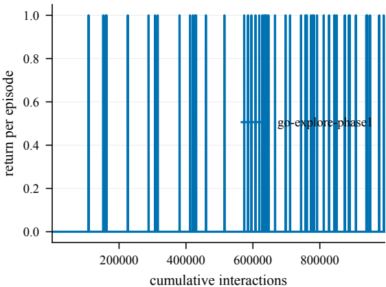
Return -- Decoys1-50@4000
