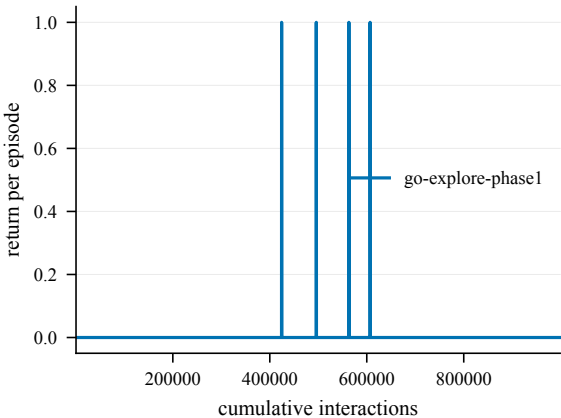
Return -- Decoys2-100@4000
