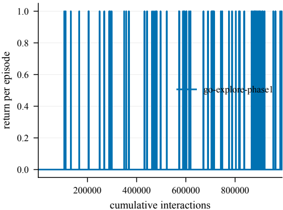
Return -- Decoys4-50@4000
