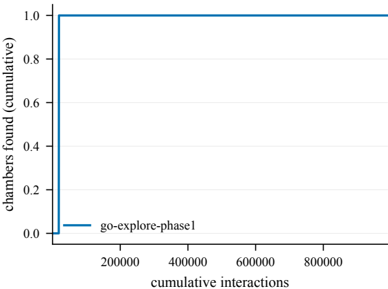
Chambers -- Decoys4-50@4002
