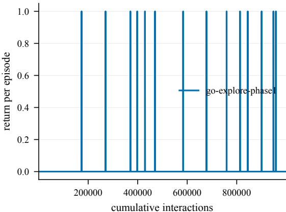
Return -- Decoys8-100@4001
