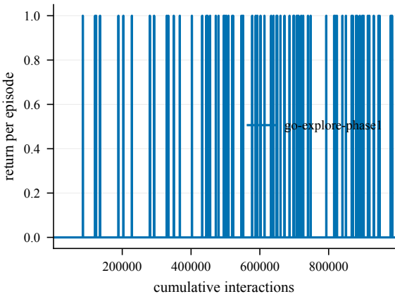
Return -- Decoys8-50@4000
