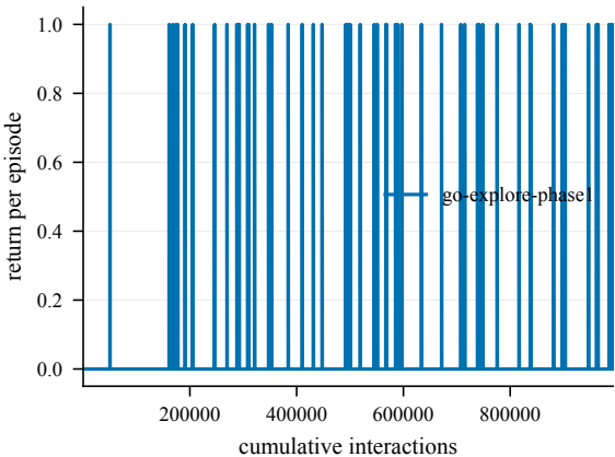
Return -- Dilution-50@4002
