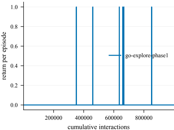
Return -- GiveUp1-100@4001
