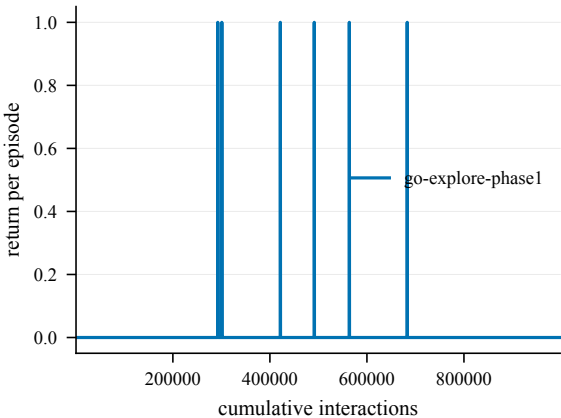
Return -- GiveUp4-100@4000
