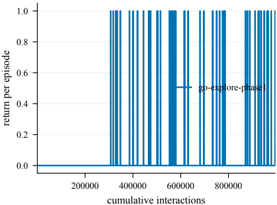
Return -- GiveUp4-50@4002
