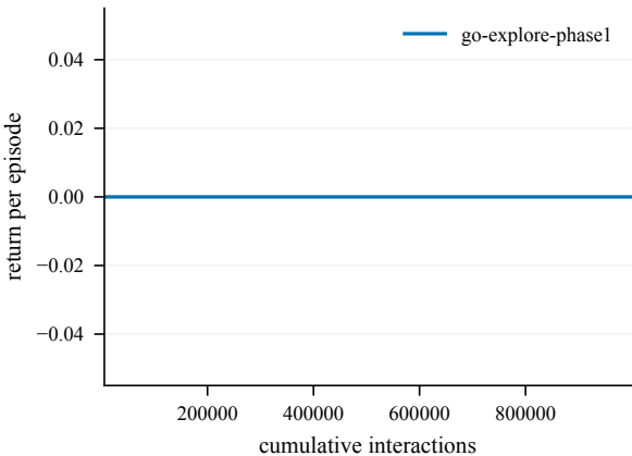
Return -- Maze-100@4000
