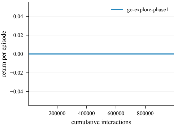
Return -- Maze-100@4001
