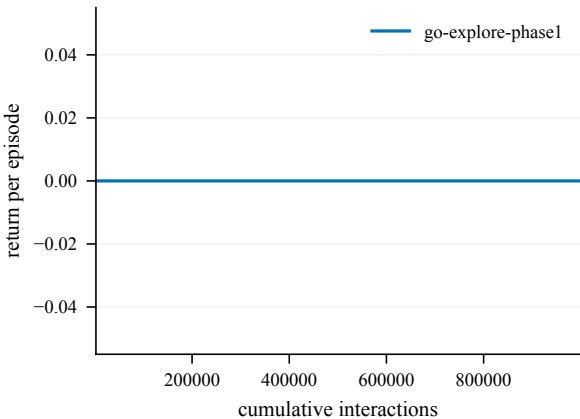
Return -- Maze-50@4002
