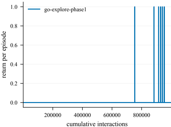
Return -- Nested1-100@4002
