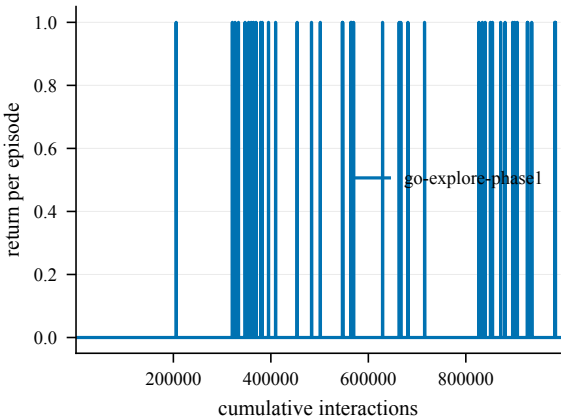
Return -- Nested2-50@4002
