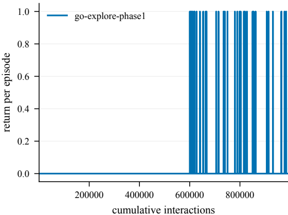
Return -- Nested3-50@4001
