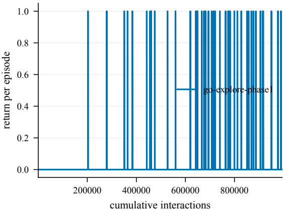
Return -- ShapeCi-50@4002
