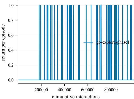
Return -- ShapeSt-50@4001
