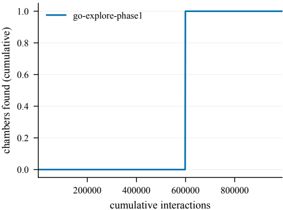
Chambers -- BankRobber@4000
