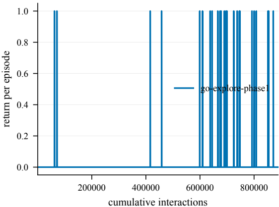
Return -- DontFall@4000
