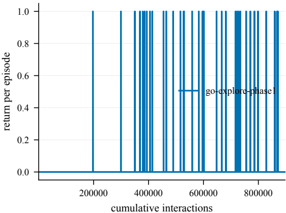
Return -- DontFall@4002
